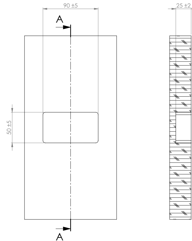
SCHNITT A-A
