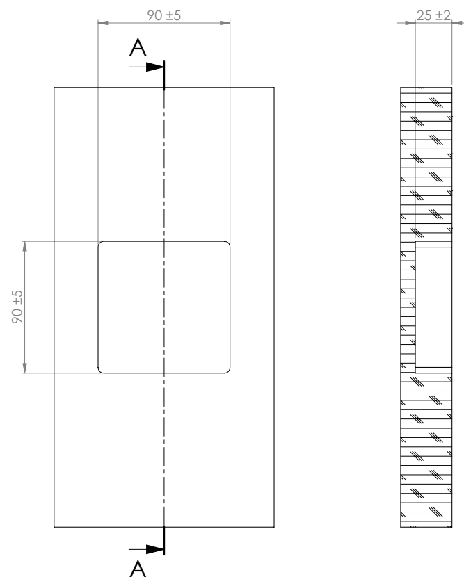
SCHNITT A-A
